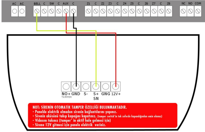
METAL PANEL ile WS-244 ve WS-249 BAĞLANTI ŞEMASI
